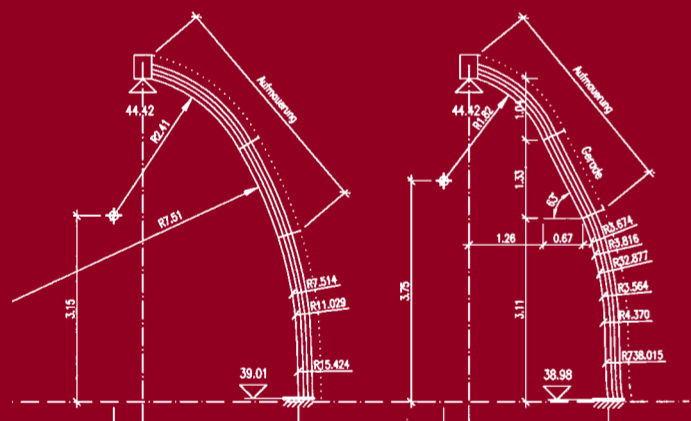
Konstrukcja żebier sklepiennych
