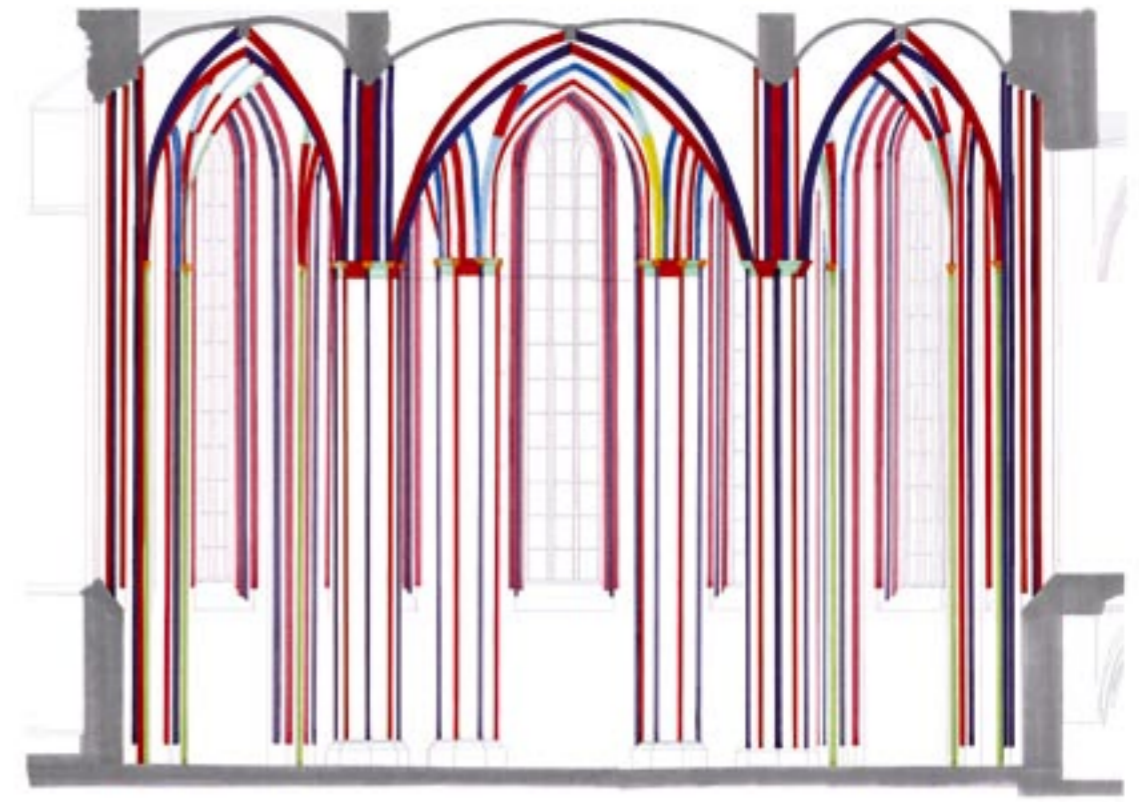
Przekrój pionowy prezbiterium z obejściem
