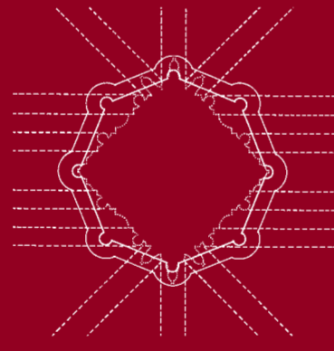
Przekrój filara
